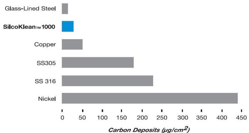
Abbildung 2: SilcoKlean®1000 Beschichtung reduziert Verkokung um das 8-fache. Datenquelle ist die Pennsylvania State University
